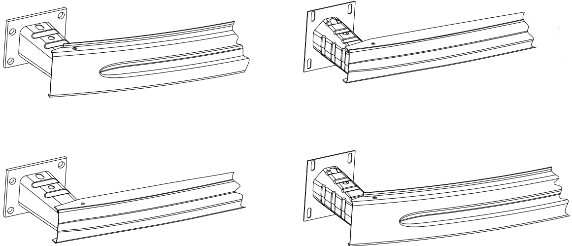
Abbildung 6.8: Varianten der CMS-Geometrie, die durch die Kombination aus jeweils zwei unterschiedlichen Geometrietemplates von Crashbox und Querträger erstellt wurden.
