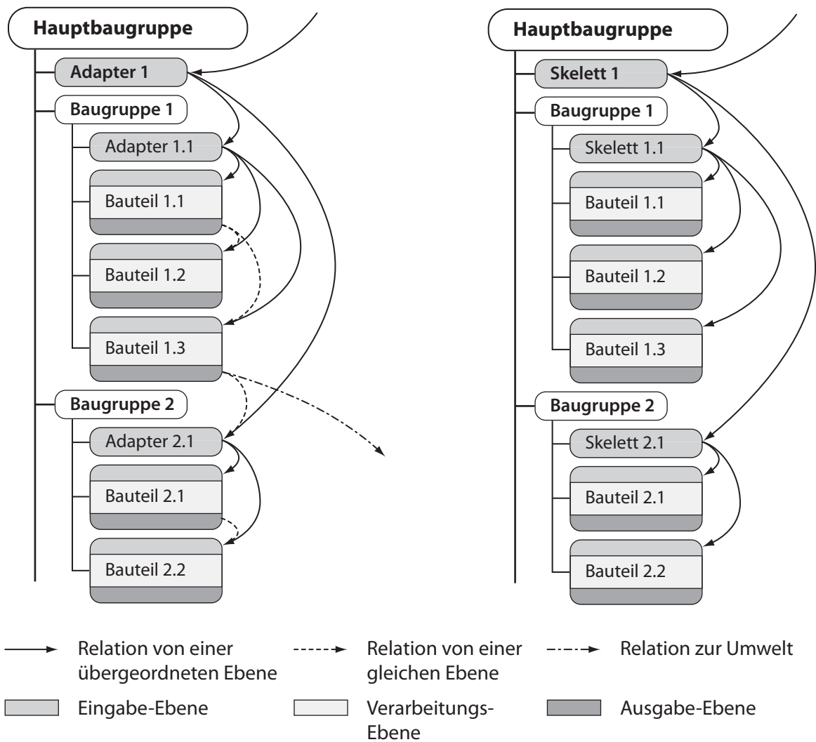
Abbildung 3.11: Verknüpfungen, die für eine Geometrieadaption innerhalb eines Matingtemplates verwendet werden (links Adaptermodelle , rechts Skelettmodelle ), nach [Bra09].
