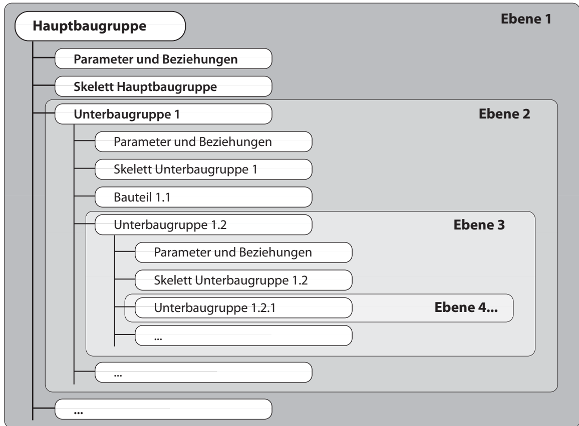
Abbildung 3.9: Typischer Aufbau einer Baugruppenstruktur, nach [HHR11].
