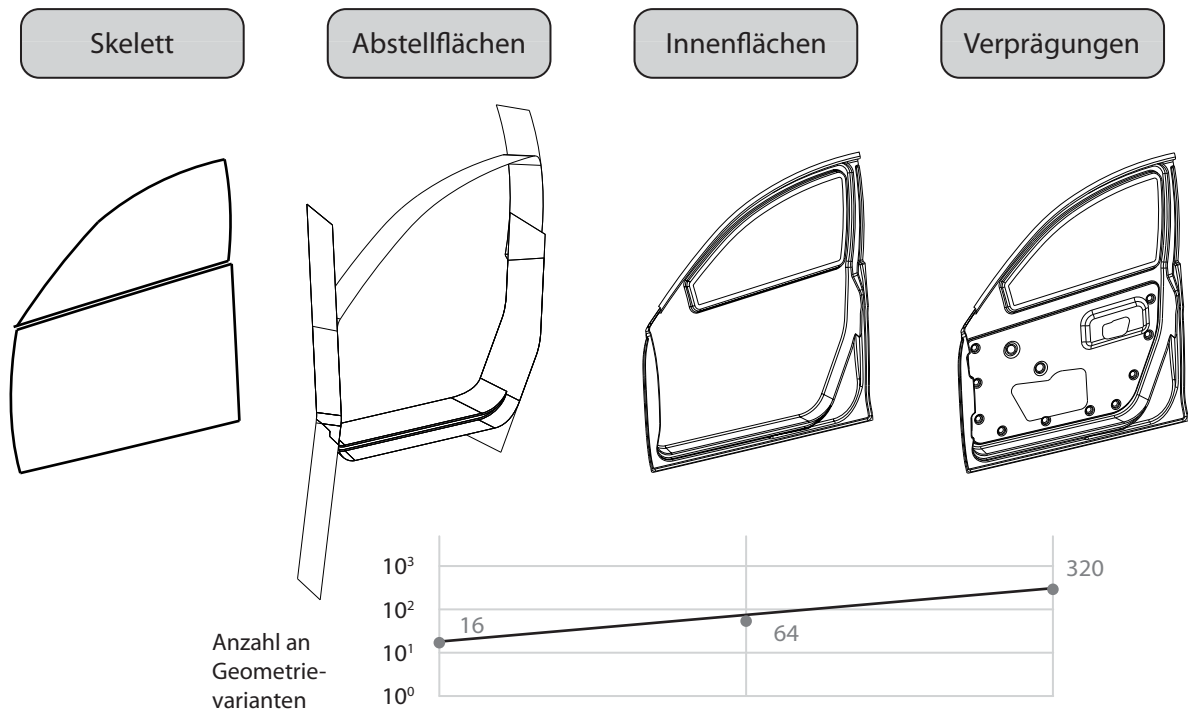
Abbildung 5.17: Abfolge der Geometriemodellierung innerhalb des Türinnenblech-Geometriemplates.
