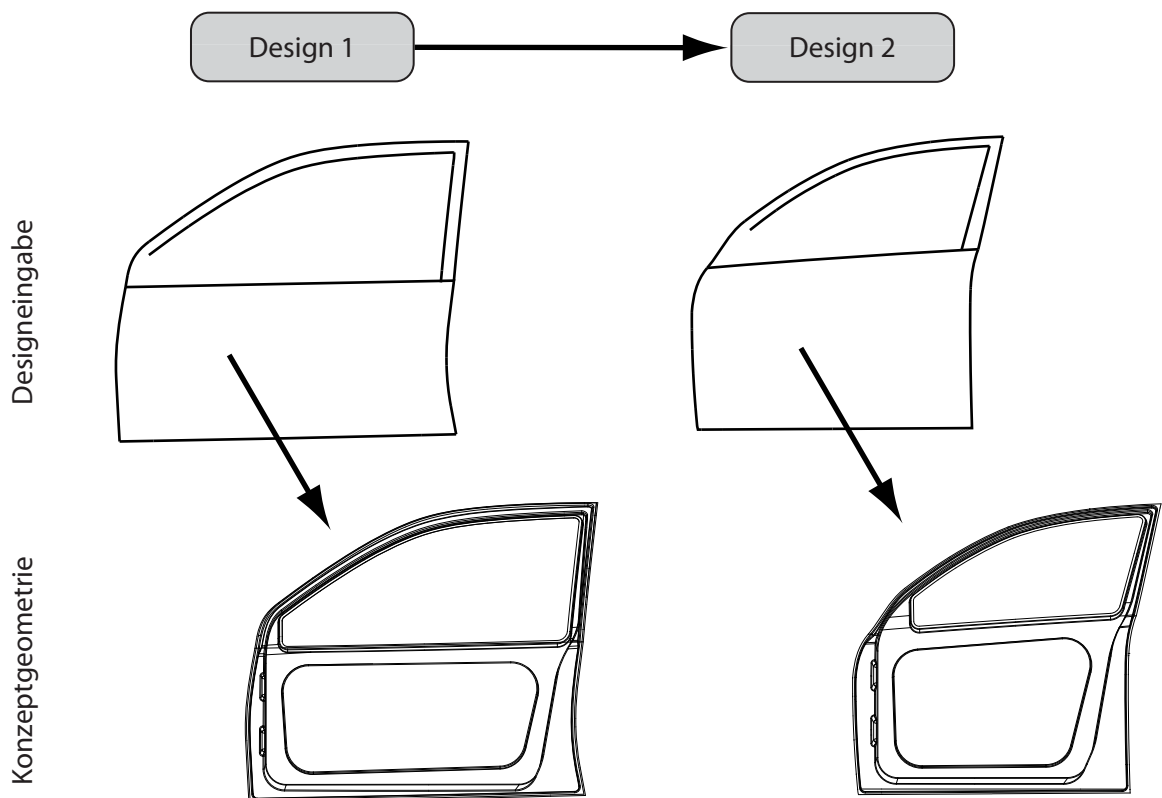
Abbildung 5.19: Anpassung der Geometrie des Türinnenblech-Geometrietemplates an ein geändertes Fahrzeugdesign.
