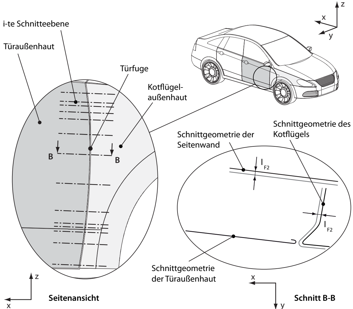
Abbildung 5.5: Lösungsraum für die Positionierung der Scharnierdrehpunkte.
