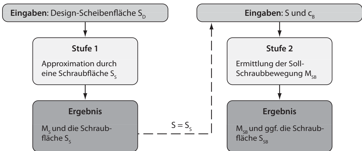
Abbildung 5.13: Schematische Vorgehensweise zur Ermittlung einer approximierten Scheibenfläche S_S und der Sollbewegung M_{SB} .
