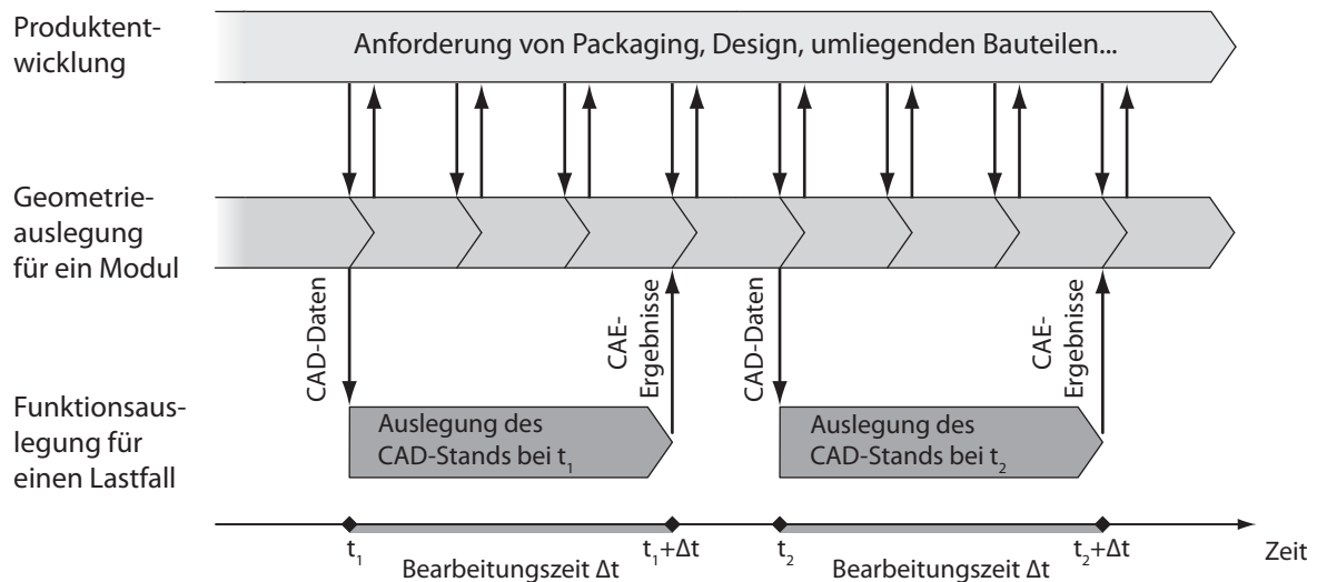
Abbildung 4.2: Parallel ablaufende Geometrie- und Funktionsauslegung in der Konzeptphase, nach [Her07] 26 .
