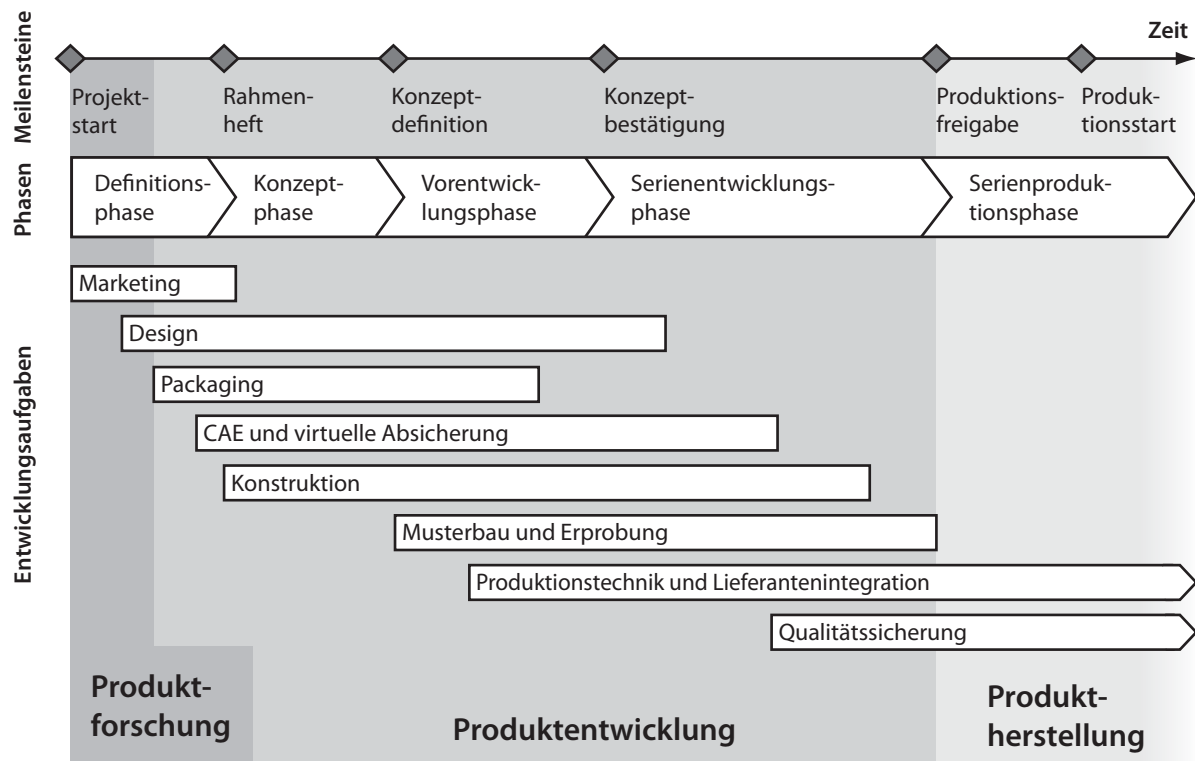
Abbildung 2.1: Exemplarischer Produktentstehungsprozess bei einer Fahrzeugneuentwicklung.
